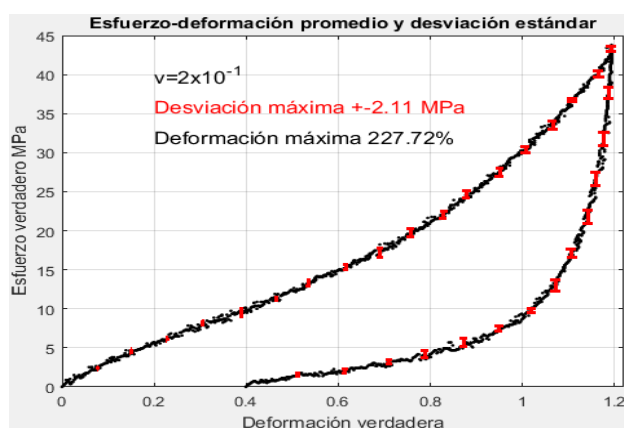
Figura 10 Curva esfuerzo-deformación promedio y barras de error expresado por su desviación estándar obtenida de la figura 8
