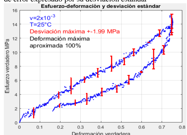
Figura 23 Curva esfuerzo-deformación promedio y barras de error expresado por su desviación estándar
