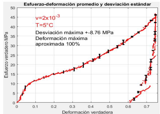
Figura 21 Curva esfuerzo deformación promedio y barras de error expresado por su desviación estándar
