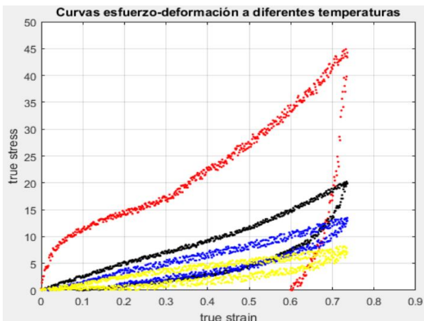
Figura 20 Cruvas esfuerzo deformación con los datos extraídos de la figura 19
