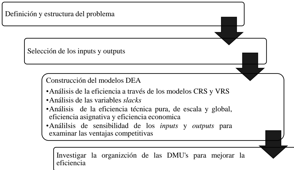
Figura 9 Metodología DEA
