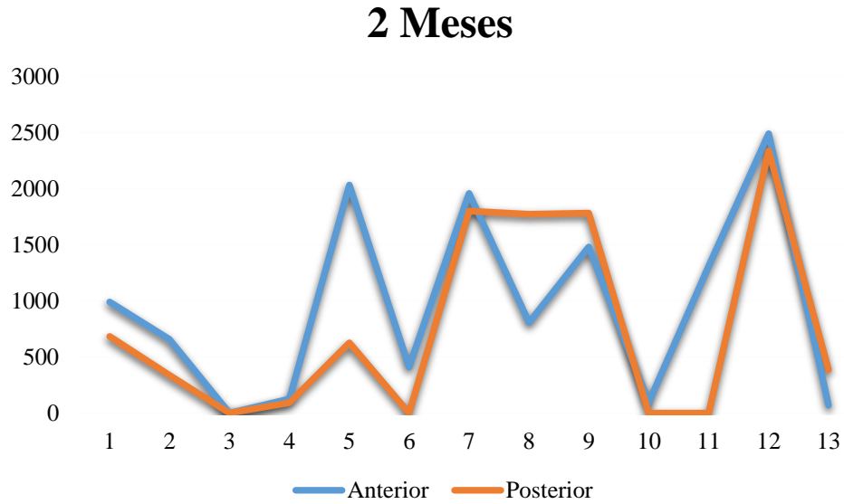
Gráfico 4.16 Análisis por series de tiempo con relación al consumo en kilowatts en 2 meses
