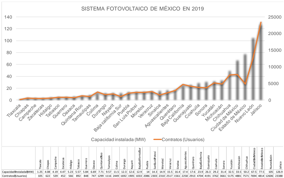
Gráfico 2.2 Sistema fotovoltaico de México en 2019
